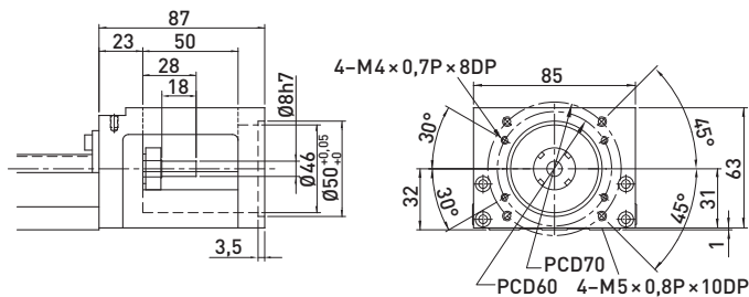
F0 motor-adapterkarima
