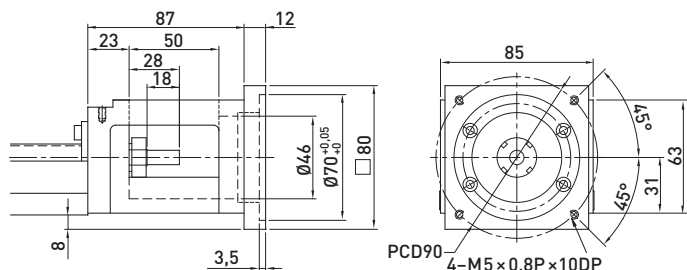
F4 motor-adapterkarima
