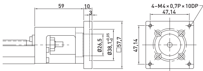
F4 motor-adapterkarima
