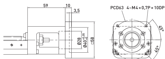
F8 motor-adapterkarima
