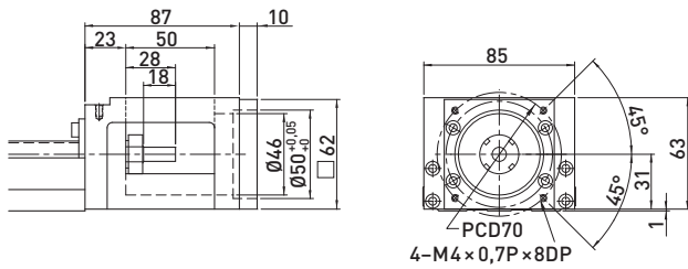
F1 motor-adapterkarima
