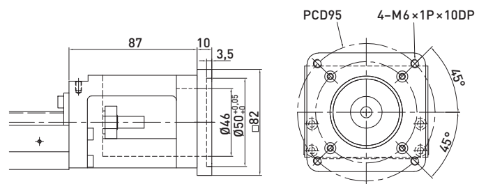
F10 motor-adapterkarima
