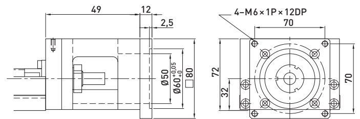
F3 motor-adapterkarima
