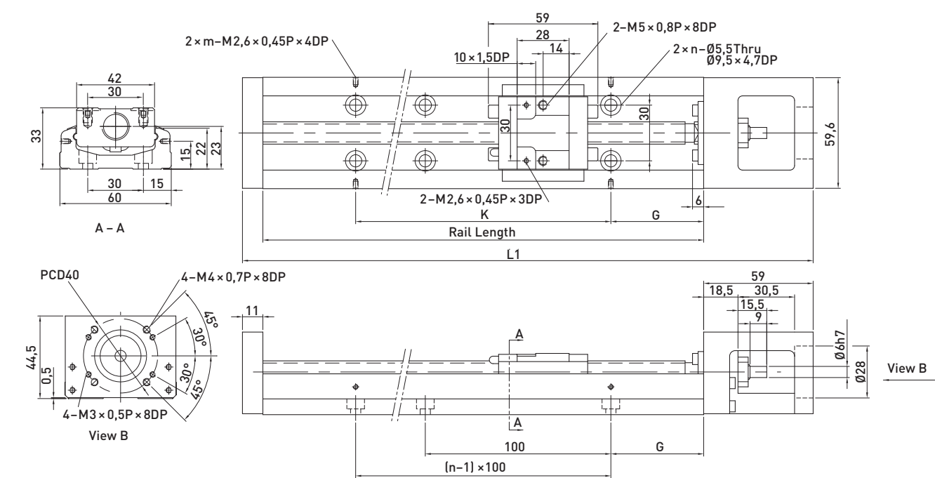
3.1.15 Borítás nélküli KK60 lineáris tengely, rövid golyóskocsi
