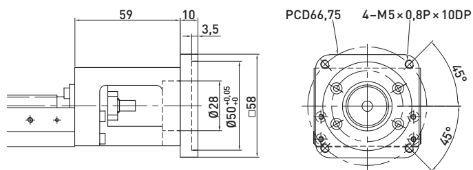
F11 motor-adapterkarima
