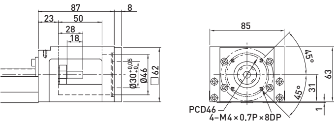
F2 motor-adapterkarima
