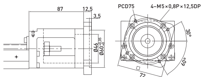
F8 motor-adapterkarima
