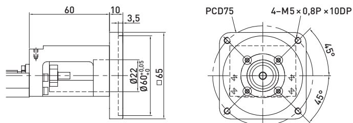
F6 motor-adapterkarima
