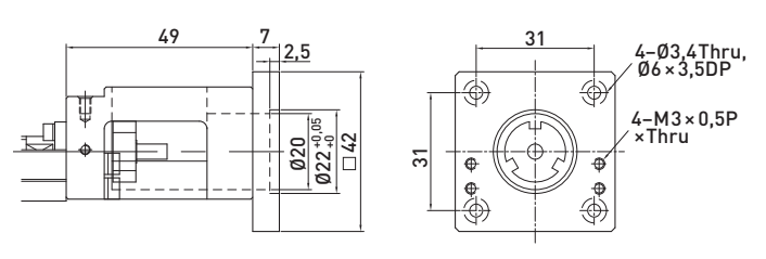
F3 motor-adapterkarima
