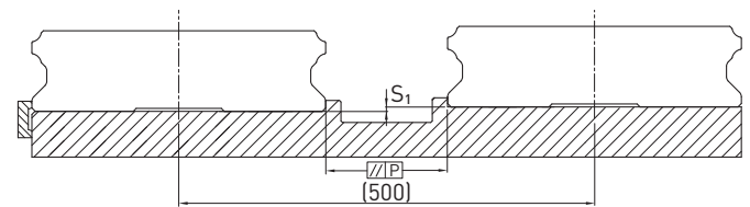
A referenciafelület párhuzamossága (P)
