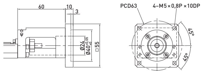
F4 motor-adapterkarima
