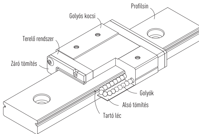
Ábra: Az MGW sorozat szerkezete
