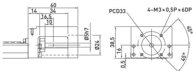
F0 motor-adapterkarima
