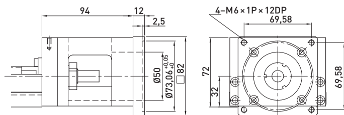
F4 motor-adapterkarima
