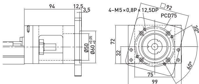
F6 motor-adapterkarima
