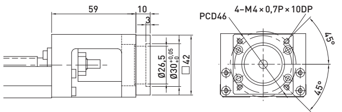
F1 motor-adapterkarima
