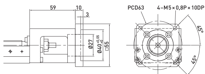
F6 motor-adapterkarima
