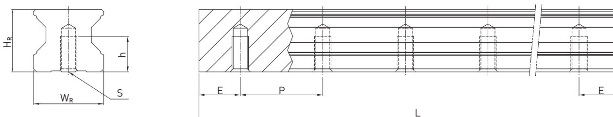
1.102 Táblázat Profilsínméretek RGR_T
