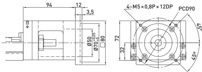
F2 motor-adapterkarima
