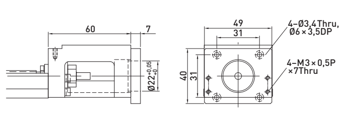
F3 motor-adapterkarima
