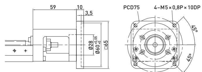
F10 motor-adapterkarima
