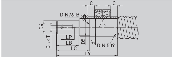
Typ E9 Csapágy: 72.. BK csapágyegységhez
