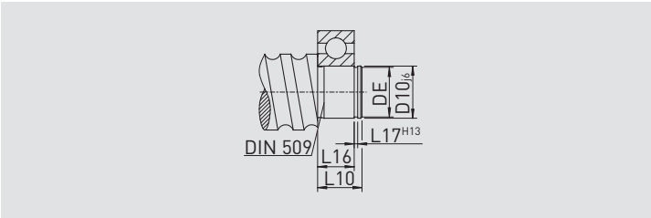
Typ E10 Csapágy: 60.. vagy 62.. gyűrűscsapágy EF, BF, FF csapágyegységhez
