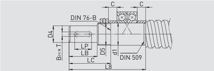
Typ E8 Csapágy: 70.. EK, FK csapágyegységhez
