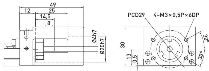
F0 motor-adapterkarima
