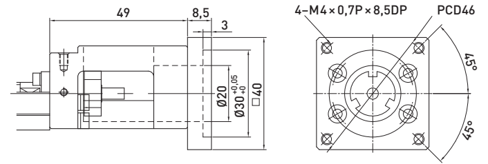
F1 motor-adapterkarima
