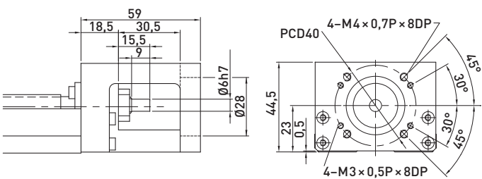
F0 motor-adapterkarima
