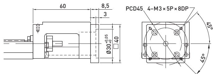
F2 motor-adapterkarima
