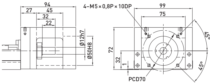
F0 motor-adapterkarima
