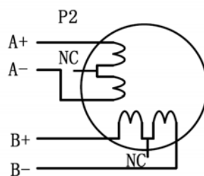
6. ábra: 6-vezetékes teljes tekercsű (nagyobb nyomaték) motor
