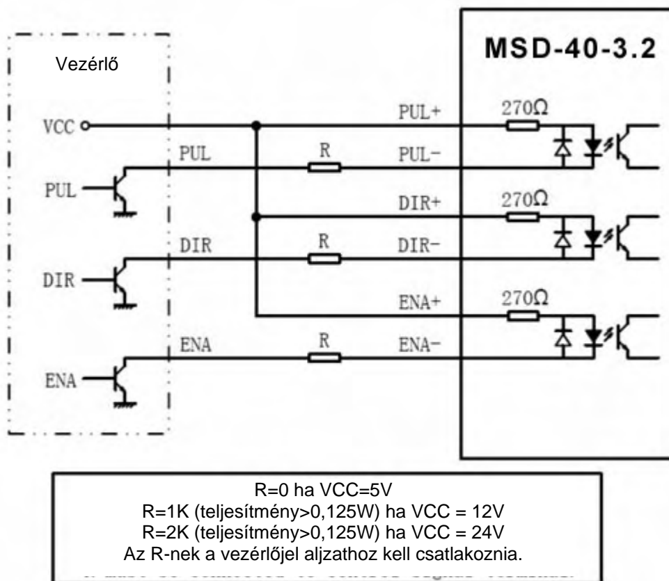
2. ábra: Csatlakozás nyitott kollektorú jelhez (közös anód)
